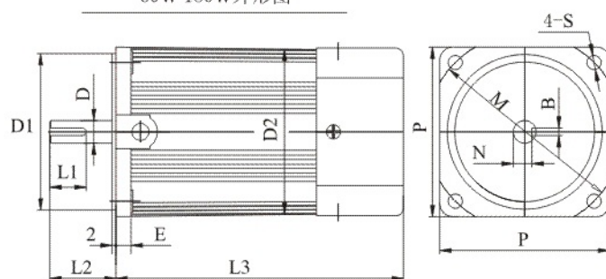
60W-180W外形图
