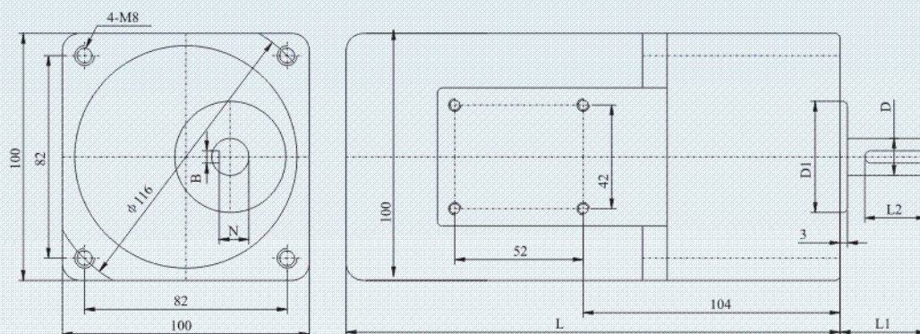
I : GK型箱体
